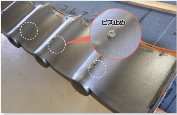
▲軒の例示工法
