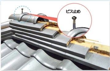
▲棟の例示工法
